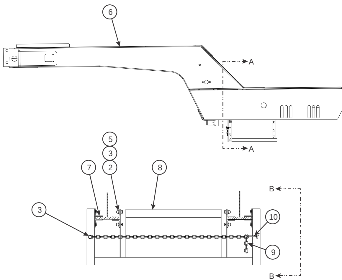
SECTION A-A
